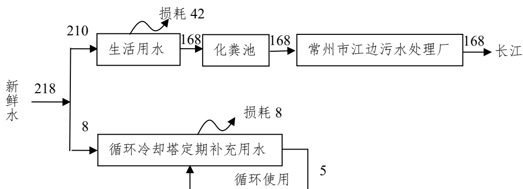
图 2-3 项目水平衡图 (t/a)
