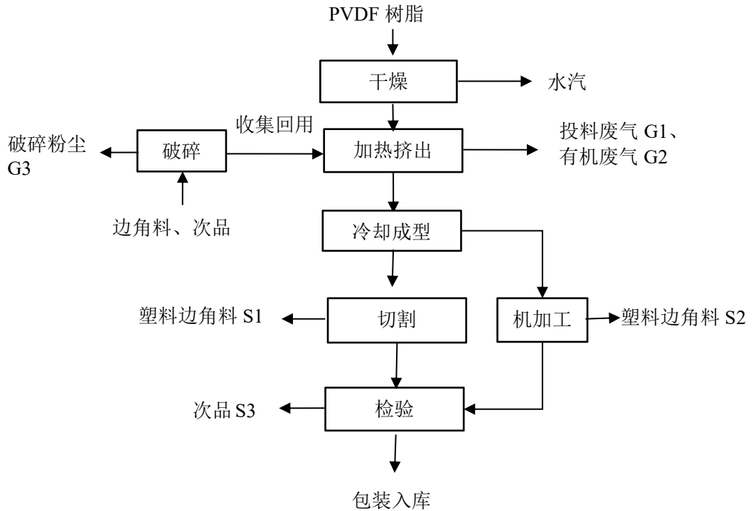
图 5-1 生产工艺流程图
